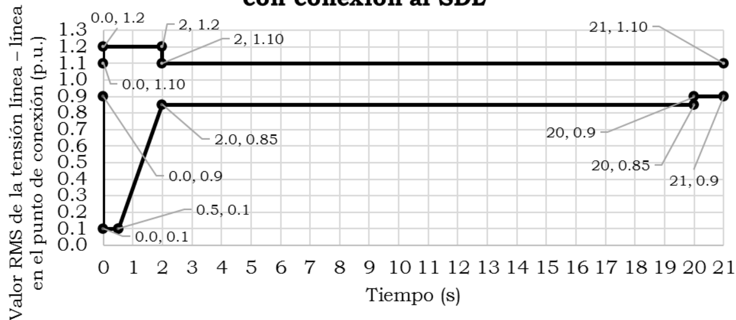
Característica de LVRT y HVRT para plantas eólicas y solares fotovoltaicas con conexión al SDL
